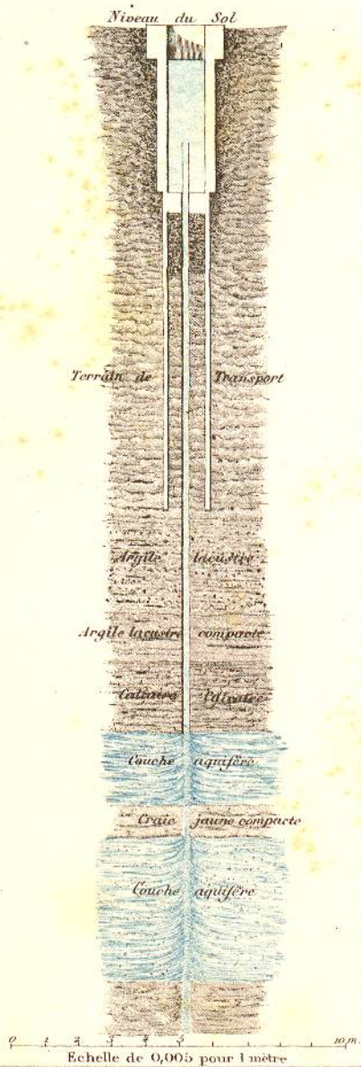
Coupe d'un puits artésien exécuté à Modène en 1850, dressée par L. SIMONIN d'après les documents locaux.
