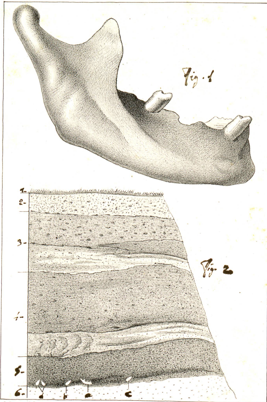
Fig. 1. mandibule semi-maculé humaine - fémur - Fig. 2. coupe géologique de la Sablière de Moulins - quignon
