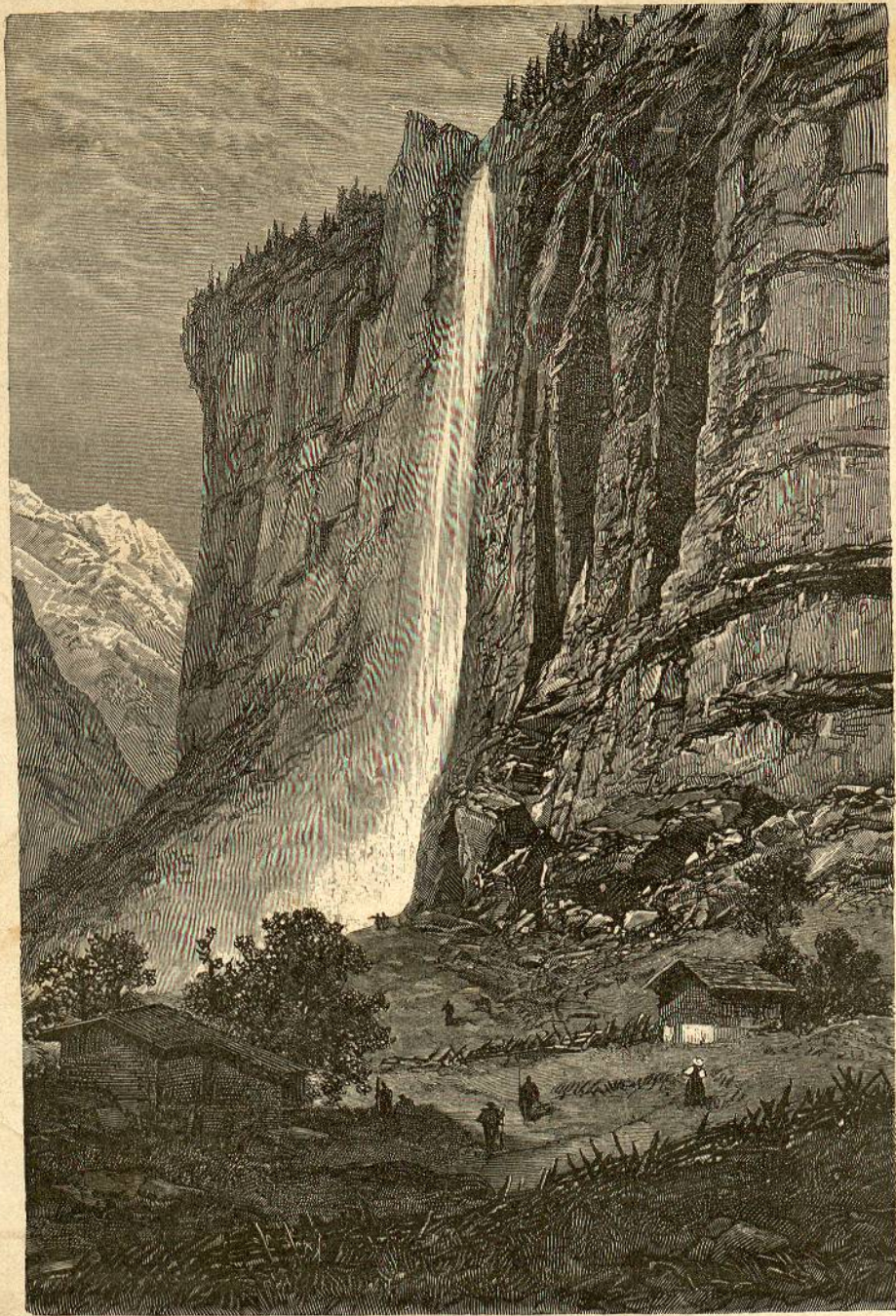
Fig. 12. — Rochers calcaires du Fletschberg et cascade du Staubach (canton de Berne), vue prise du chemin d'interlaken à la Yungfrau, d'après Rémond.
